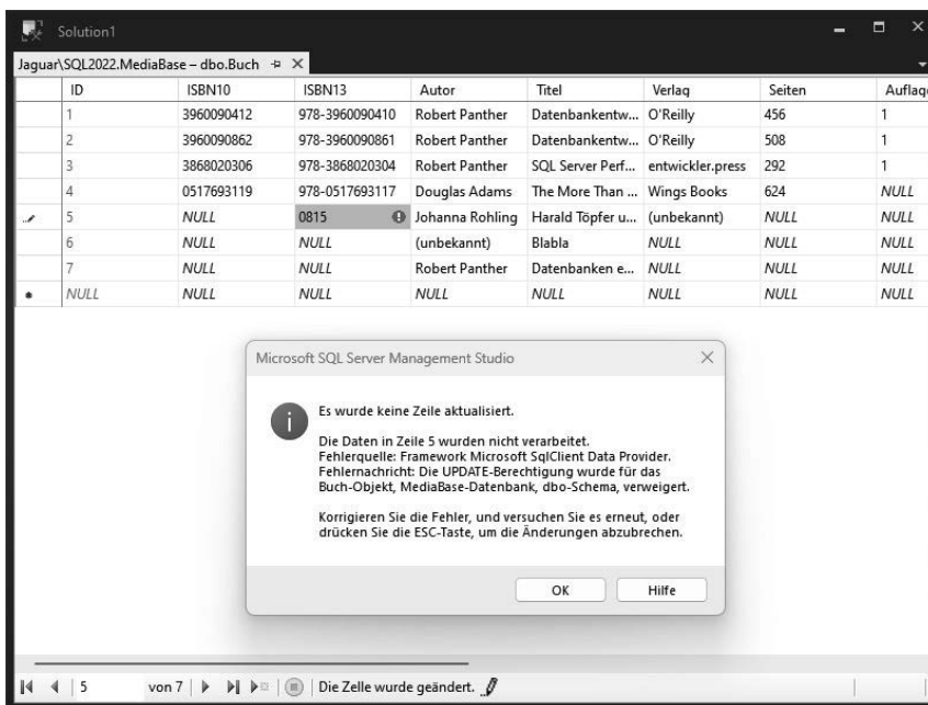
Abbildung 12.7: Fehlende Schreibrechte
