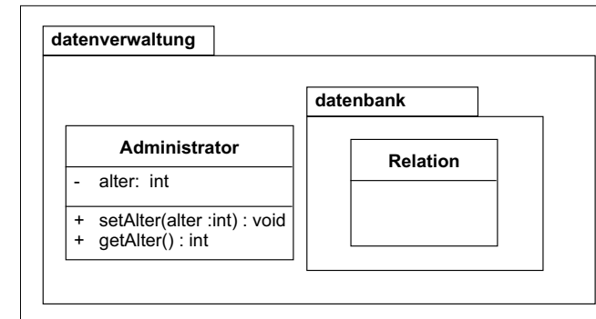
Abbildung 7.6 Beispiel eines Paketdiagramms
