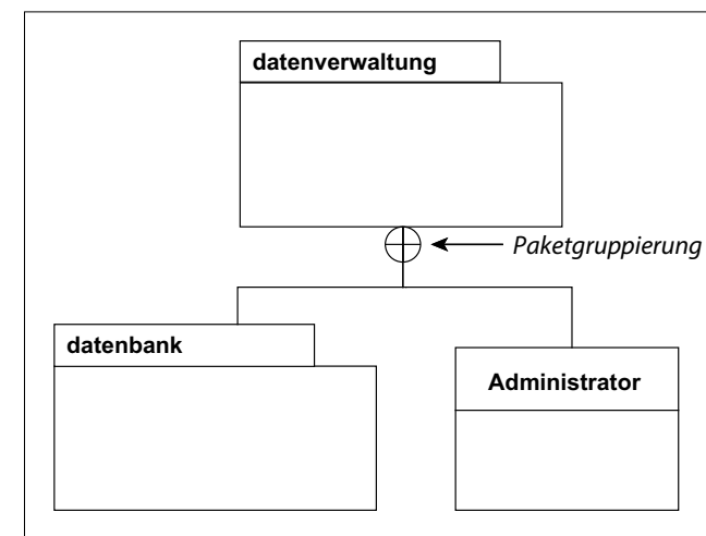
Abbildung 7.3 Gruppierung von Elementen in einem Paket
