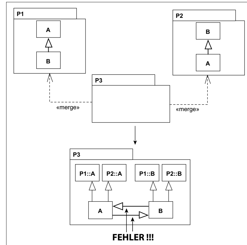
Abbildung 7.20 Gefahr der Merge-Beziehung
