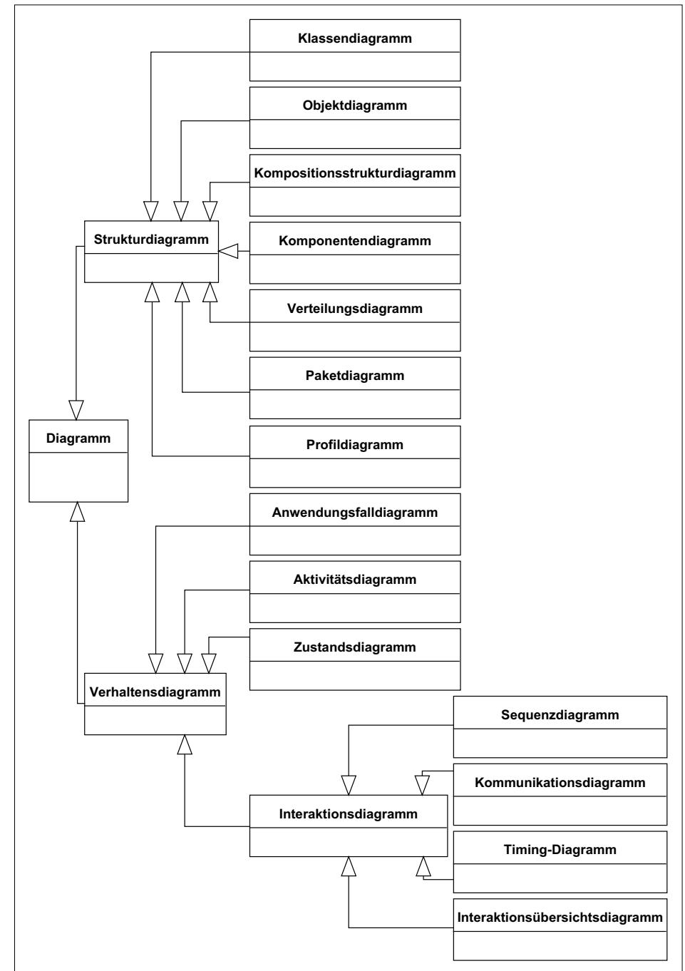
Abbildung 1.1 Übersicht über die UML-Diagramme
