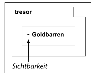
Abbildung 7.5 Sichtbarkeit eines Paketelements
