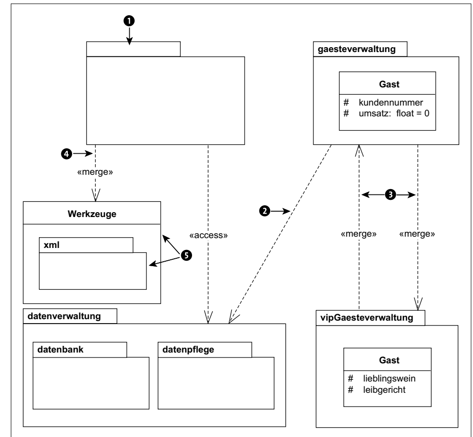
Abbildung 7.22 Ein fehlerhaftes Paketdiagramm
