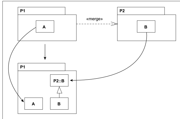
Abbildung 7.14 Merge zweier Pakete mit unterschiedlichen Elementen
