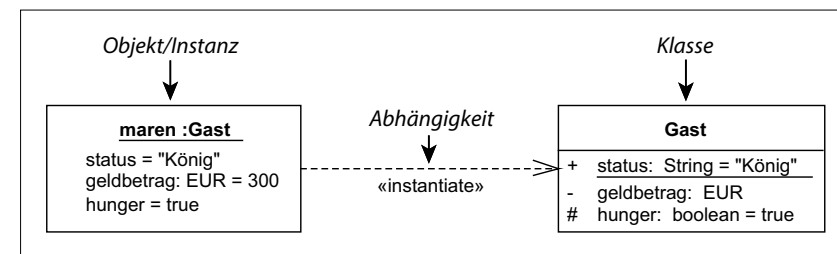
Abbildung 3.4 Instanziierung einer Klasse
