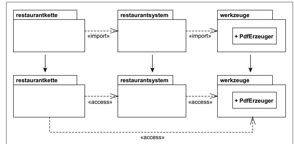
Abbildung 7.11 Umwandlung von <<import>> in <<access>>
