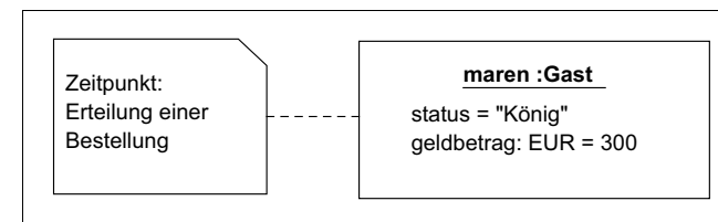
Abbildung 3.3 Unvollständige, aber zulässige Objektspezifikation
