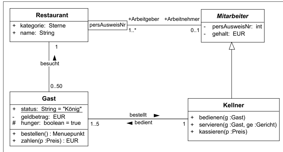
Abbildung 3.7 Klassendiagramm als Grundlage für ein Objektdiagramm
