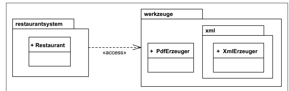
Abbildung 7.12 Beispiel für einen Paket-Import
