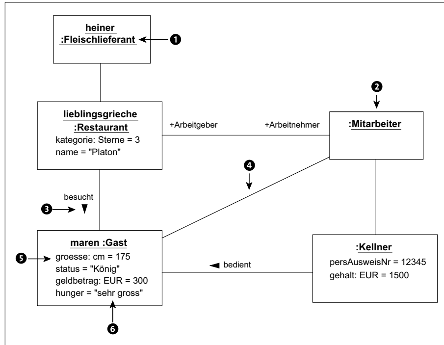
Abbildung 3.9 Mögliche Fehler in Objektdiagrammen
