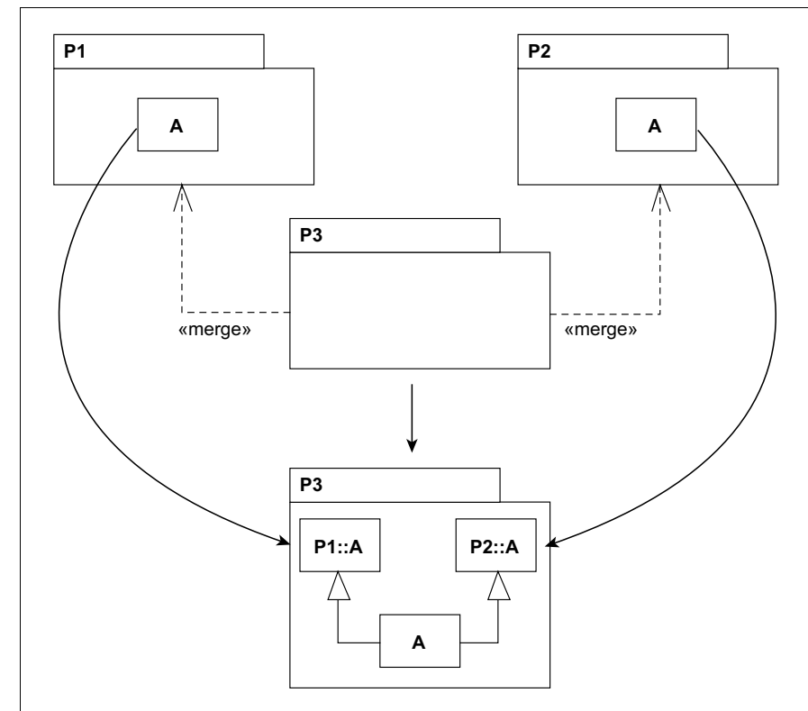
Abbildung 7.16 Ein leeres Paket mergt Elemente mit demselben Namen.
