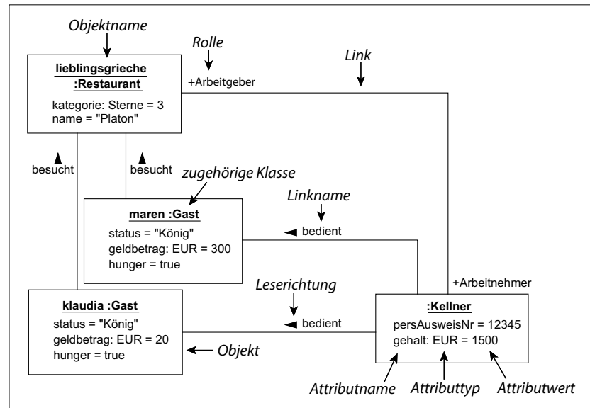
Abbildung 3.1 Notationselemente von Objektdiagrammen
