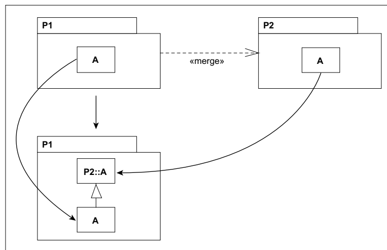
Abbildung 7.15 Merge von Elementen mit demselben Namen
