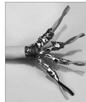
Abbildung 2.5 Netzwerk-Kabel SF/FTP nach Cat. 7
