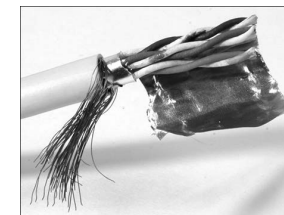
Abbildung 2.18 Freigelegte Adernpaare
