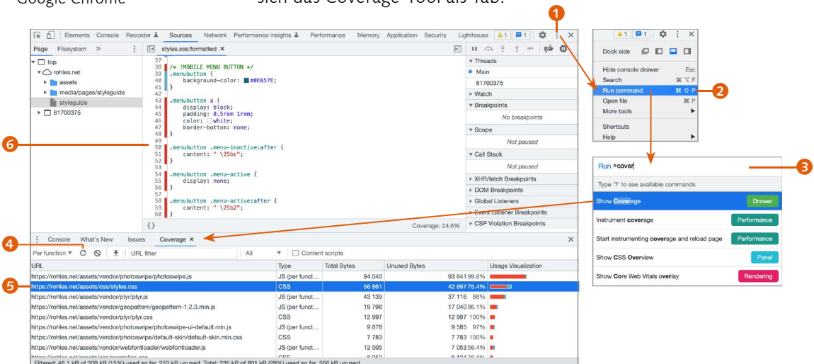
Abbildung 9.8 H Coverage-Tool in den Entwicklungswerkzeugen von Google Chrome
