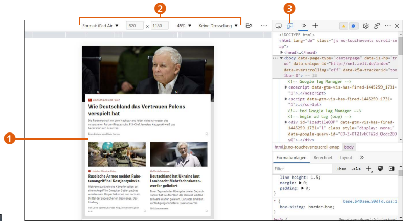
Abbildung 9.2 E Testen des Responsive Designs mit Hilfe von Chrome
