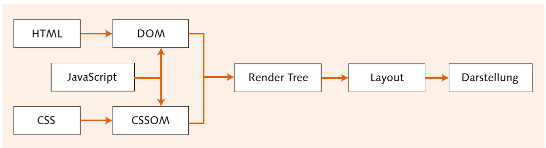
H Abbildung 9.10 Rendering-Prozess des Browsers
