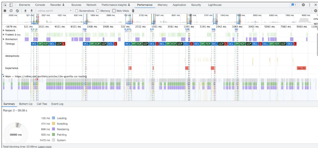
H Abbildung 9.7 Beispiel aus dem Performance-Tab in den Entwicklungswerkzeugen von Google Chrome
