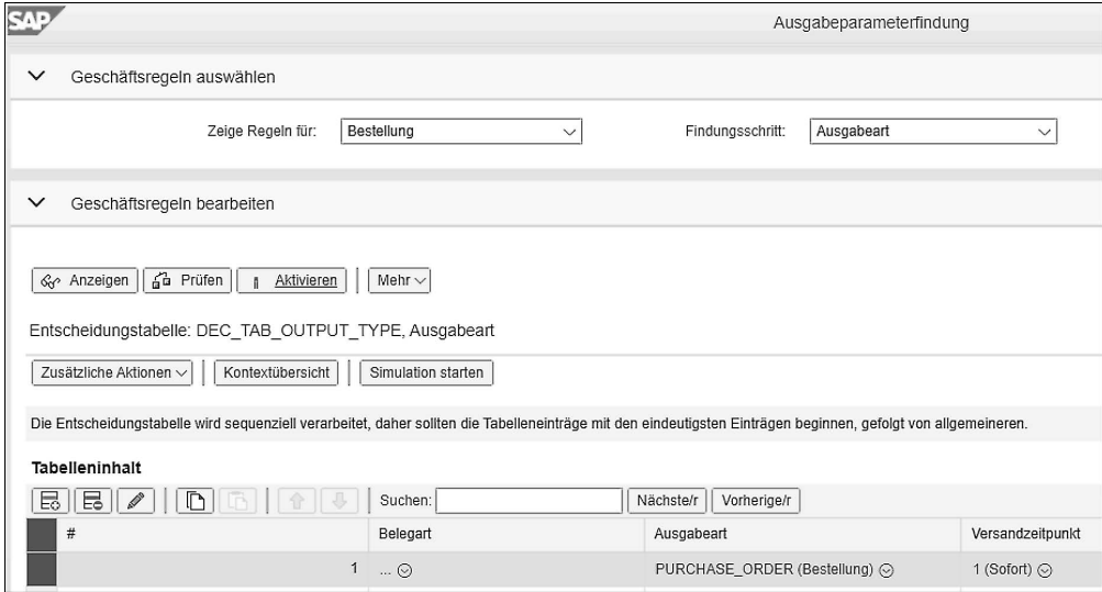
Abbildung 2.29 Versandzeitpunkt »1 (Sofort)«
