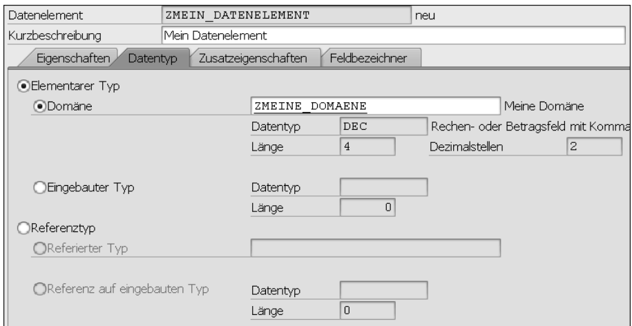
Abbildung 3.6 Datentyp eines Datenelements
