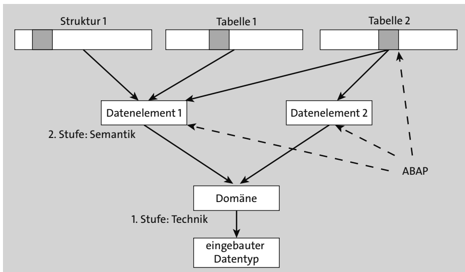
Abbildung 3.2 Das zweistufige Domänenprinzip
