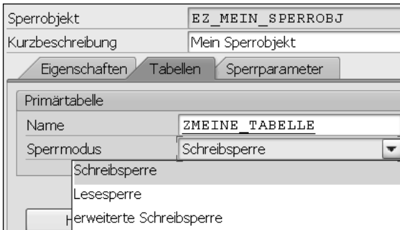
Abbildung 3.42 Sperrmodi eines Sperrobjekts
