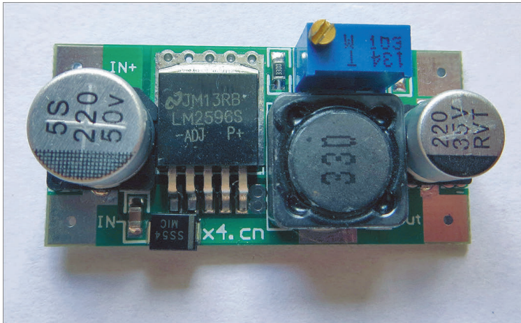
Abbildung 11.9 Fertigmodul LM2596S
