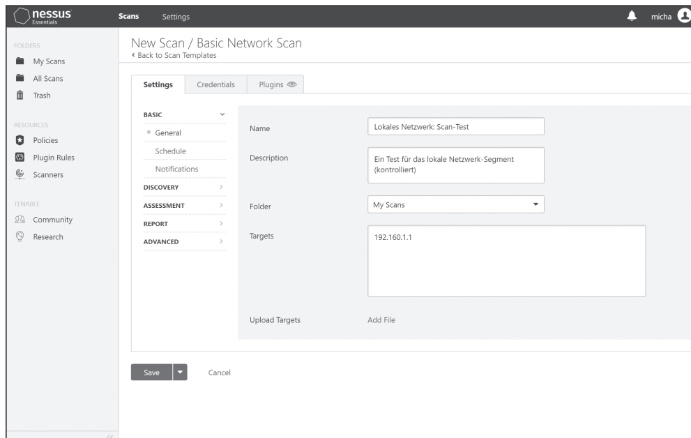
Abbildung 1.1: Wie Sie im Tool Nessus einen IP-Bereich eingeben, den Sie scannen möchten
